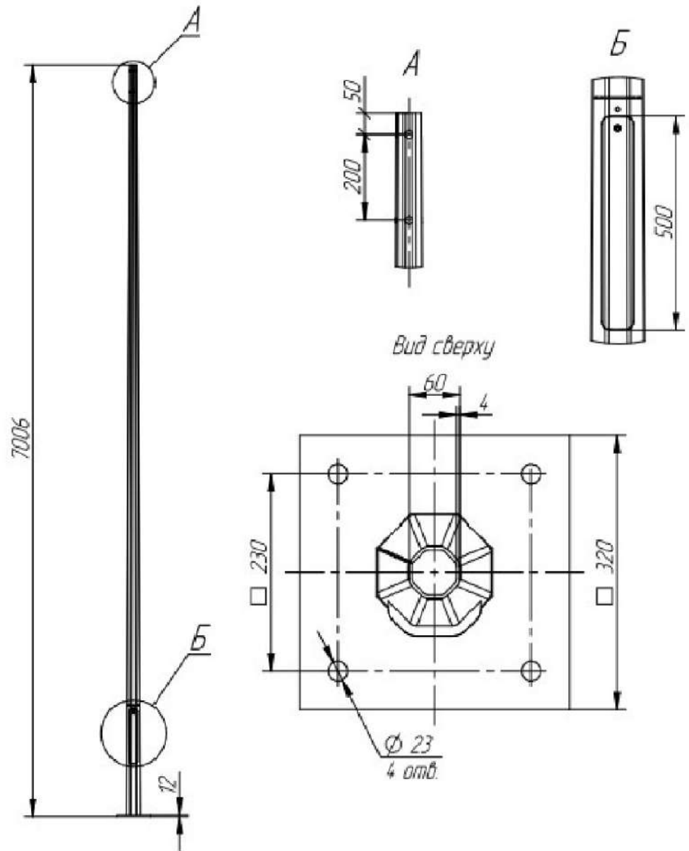
Опора
