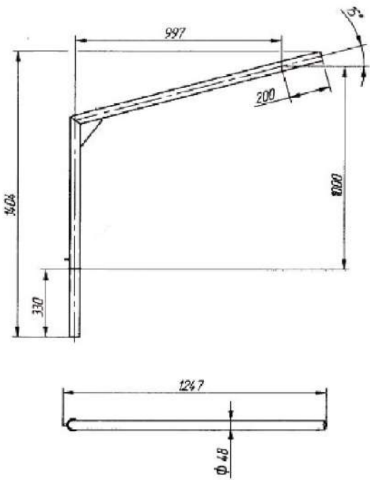
Кронштейн
